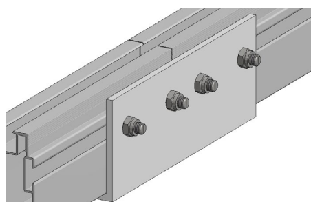
SPOJKA - NOSIČ 75
