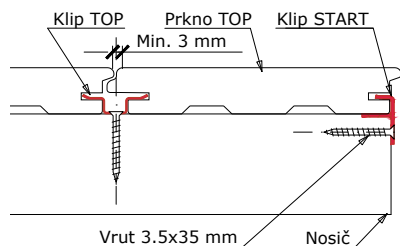
Obr. 3 Kotvení terasových prken TOP pomocí nerezových klipů a vrutů
