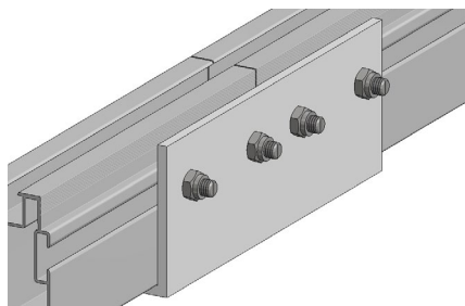
SPOJKA - NOSIČ 75
