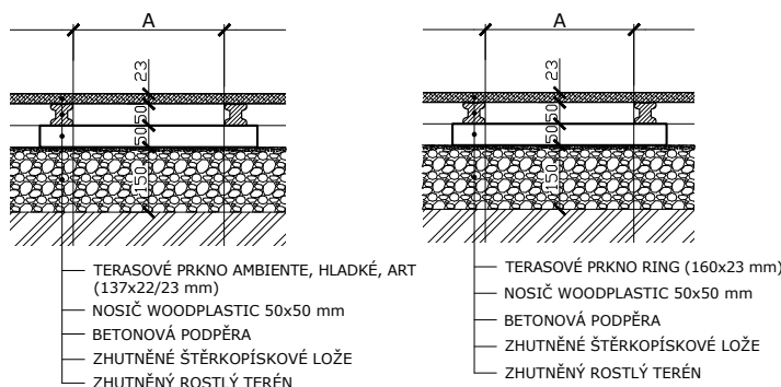
Obr. 1 Skladba terasy včetně výšek při použití nosičů WoodPlastic® 50 x 50 mm
