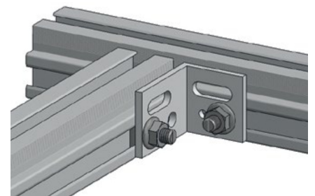
AL - SPOJOVACÍ ÚHELNÍK
